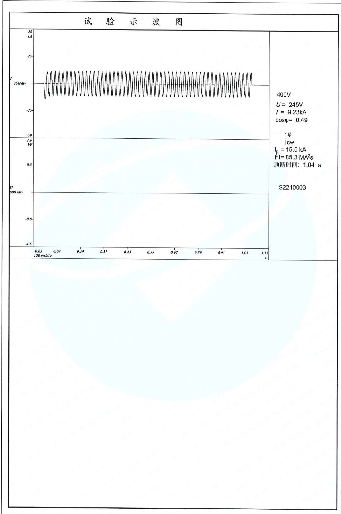
中性母线短路耐受强度验证试验示波图
