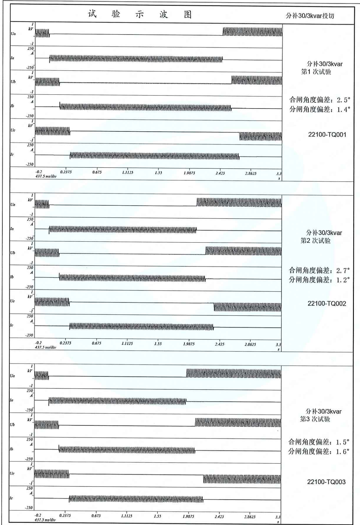
分补 30/3kvar 电容器示波图
