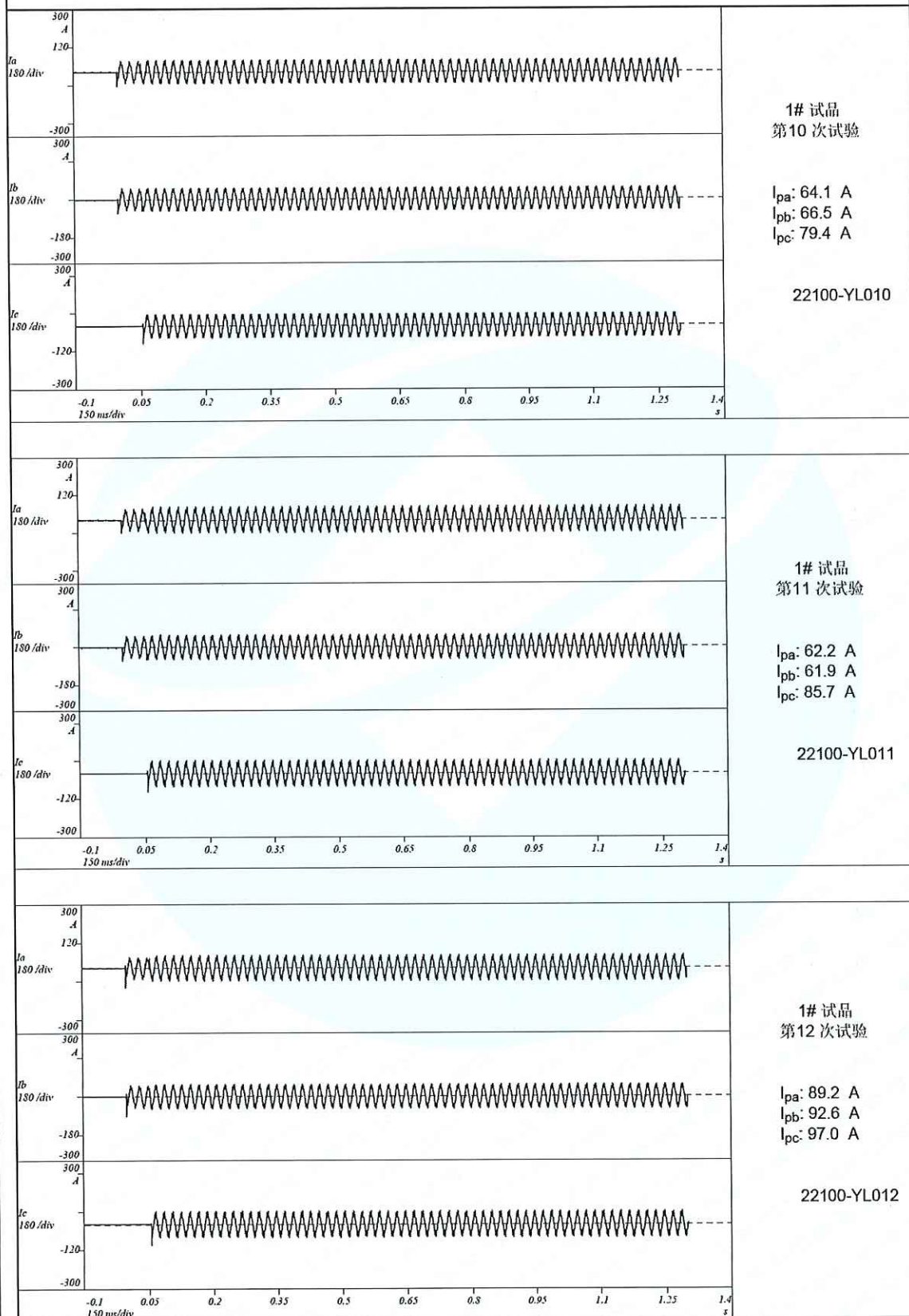
试 验 示 波 图
