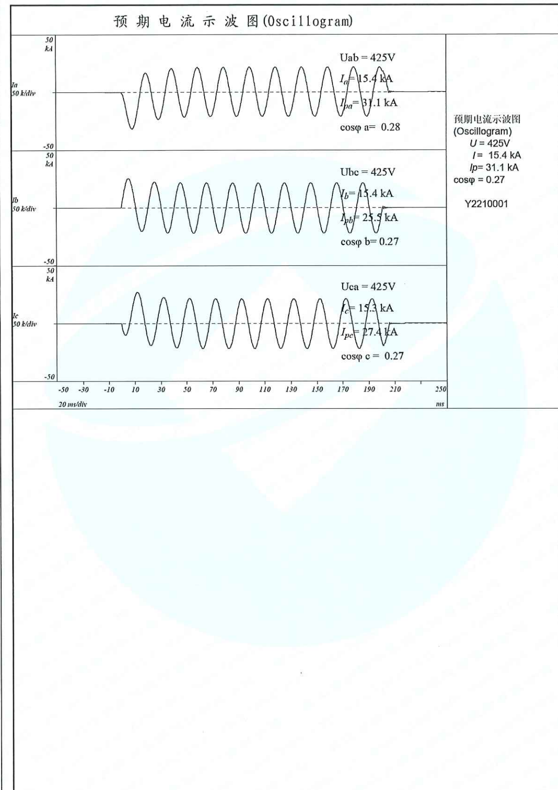
附图 10.15 短路试验示波图
