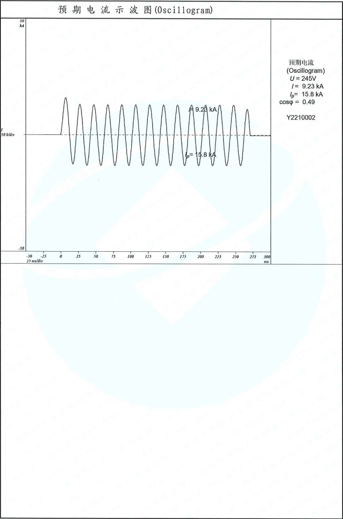
9kA 预期示波图
