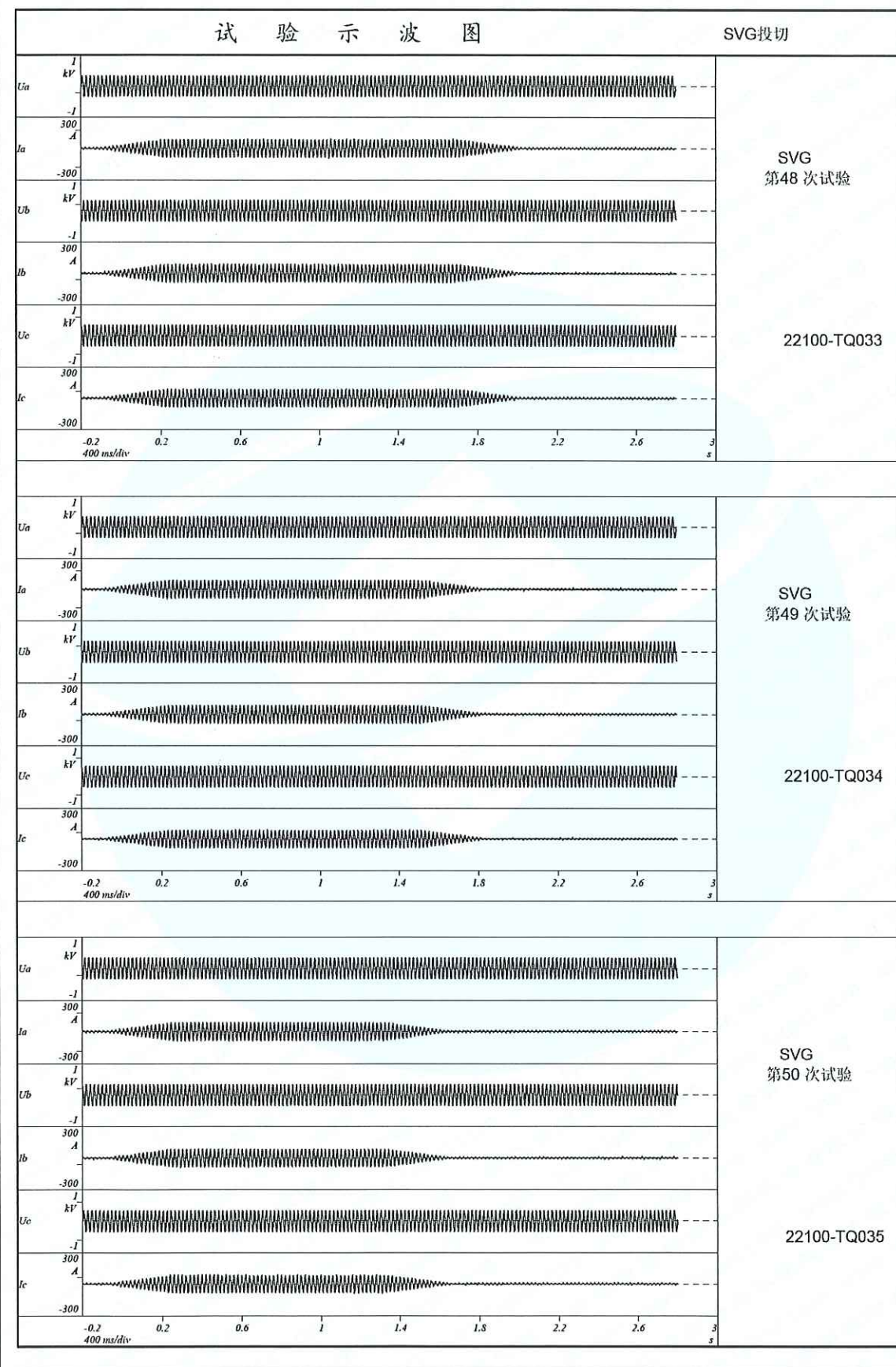
SVG 投切示波图
