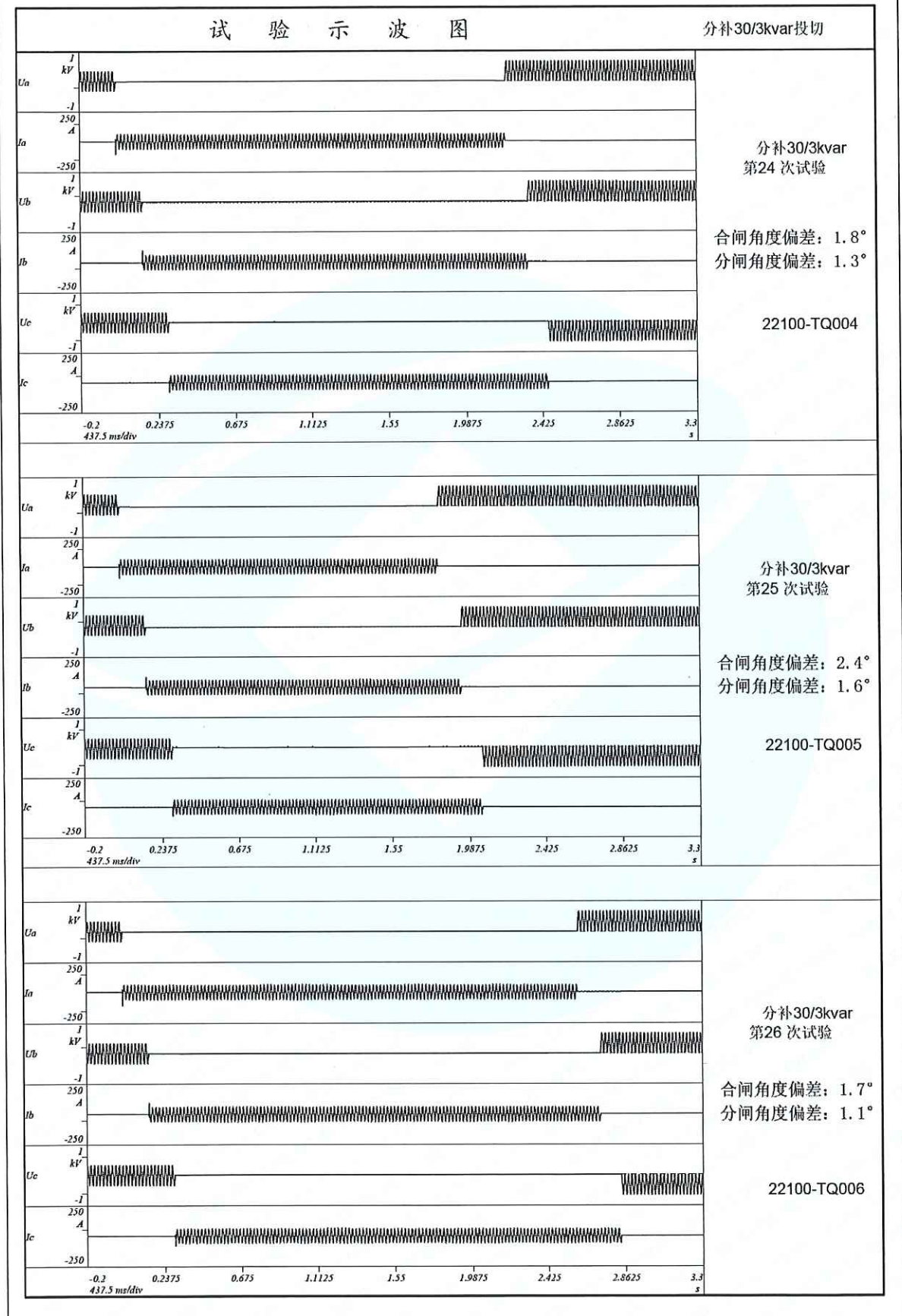
分补30/3kvar 电容器示波图
