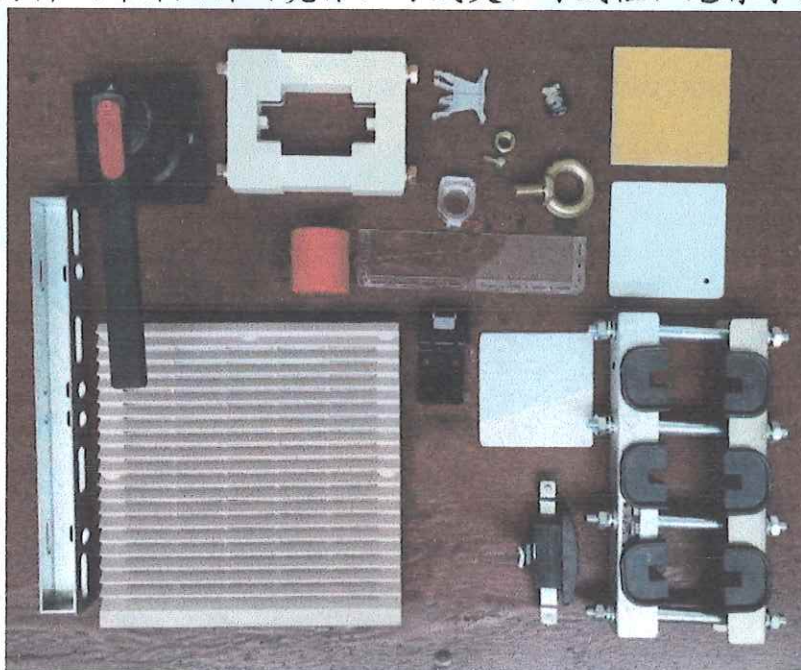
材料及部件照片（壳体、母线夹、母线框、绝缘子）
