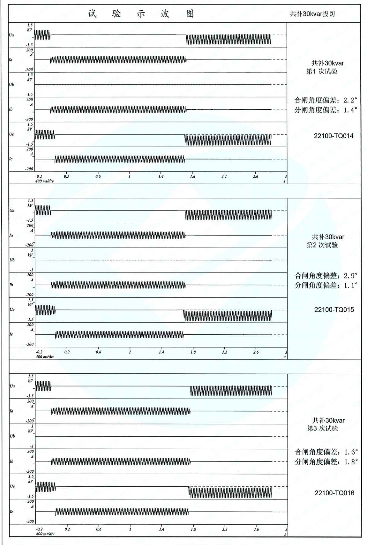
共补 30kvar 电容器示波图
