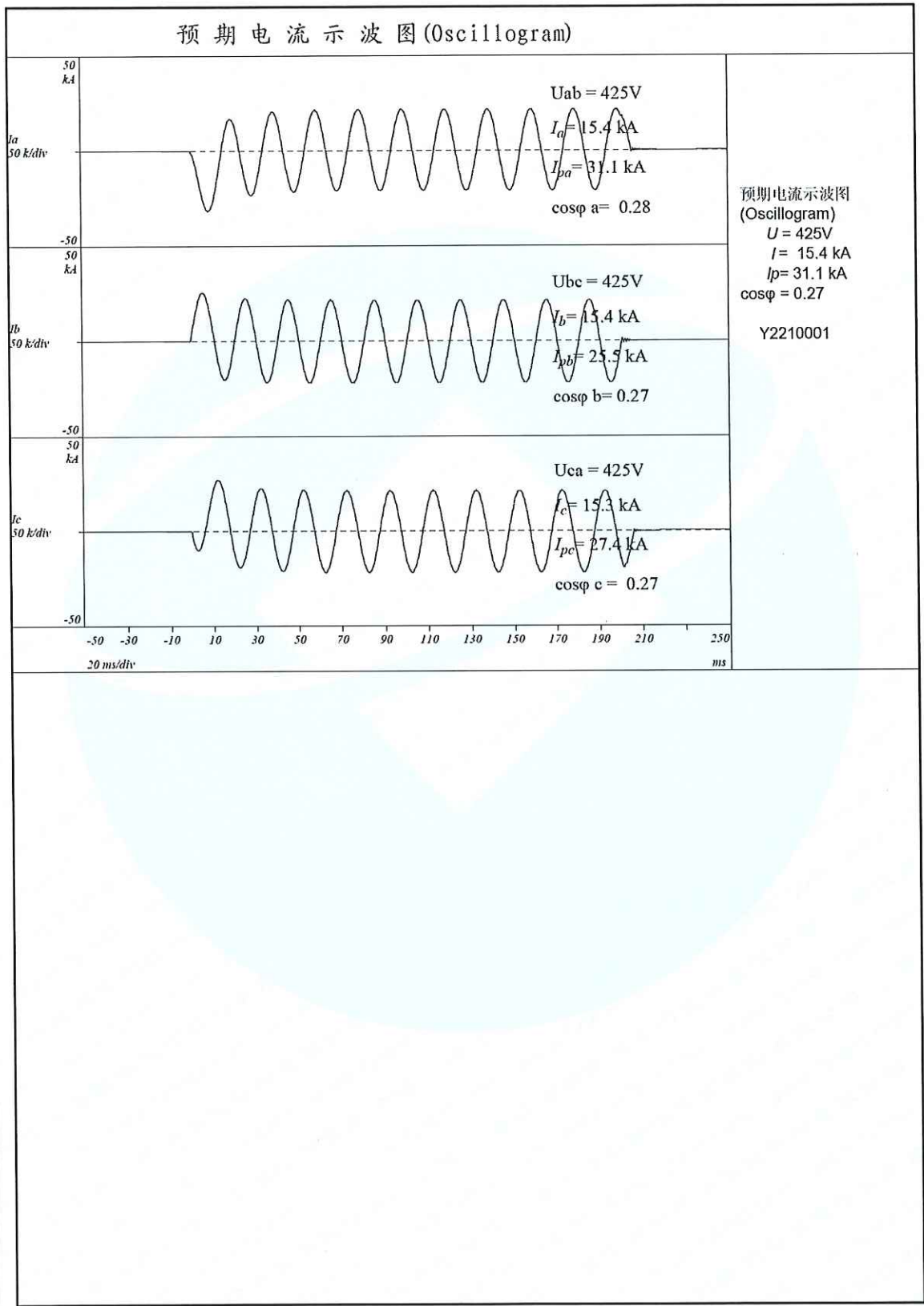
15kA 预期示波图
