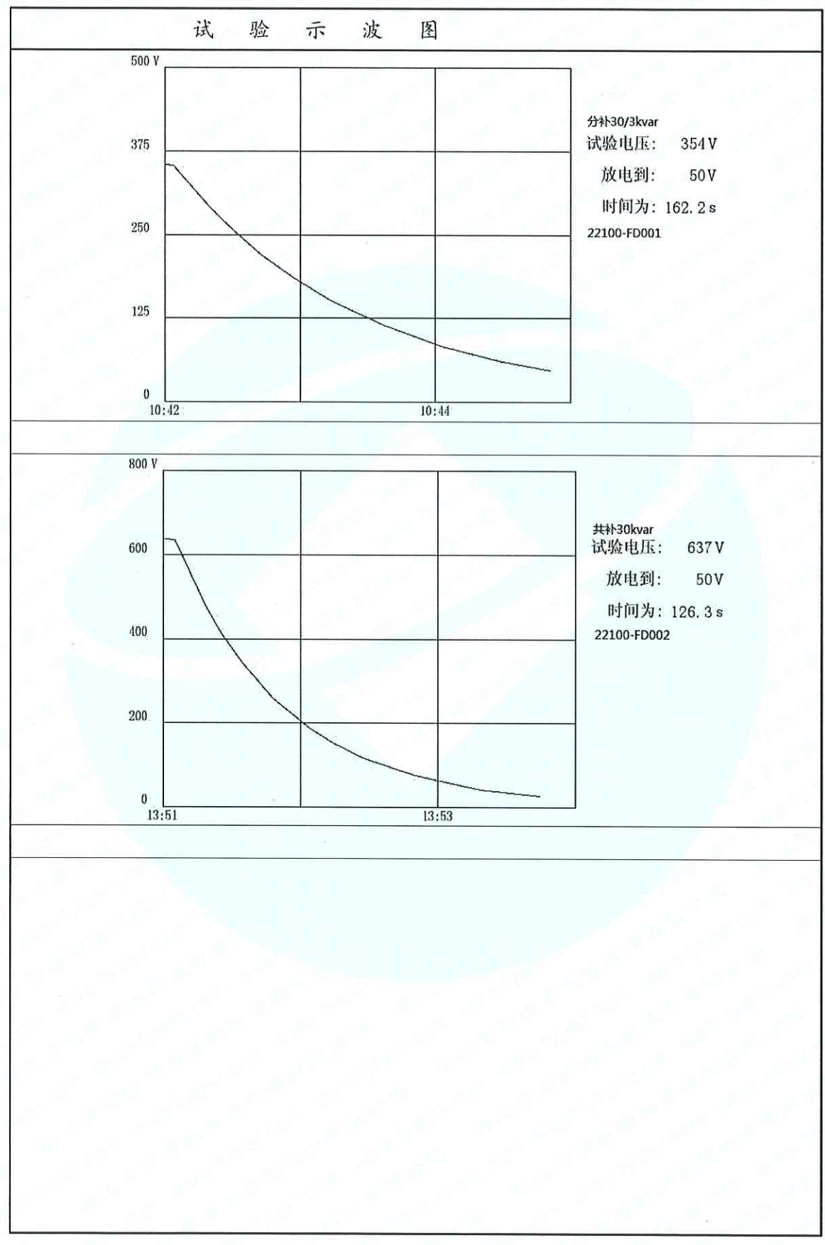
附图 10.20.5 电容器放电试验示波图
