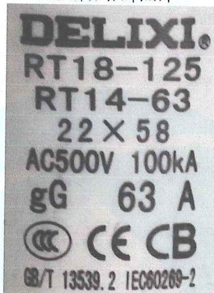
熔断器铭牌照片
