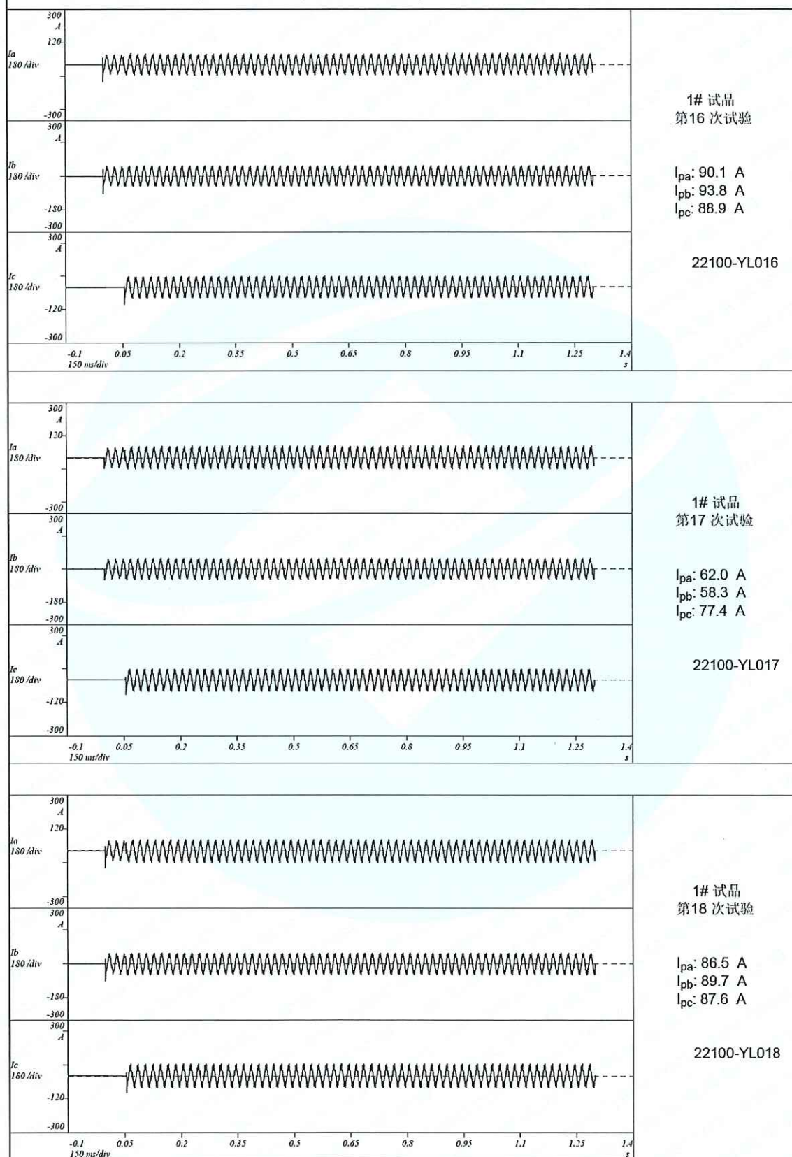
试 验 示 波 图
