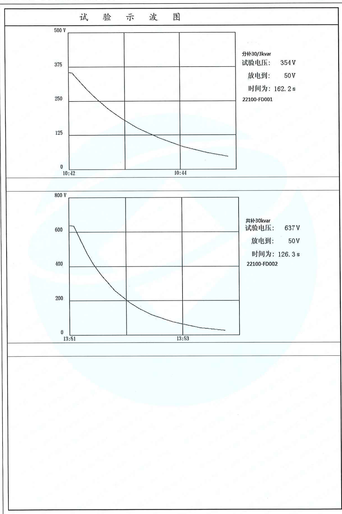
附图 9.16 电容器放电试验示波图
