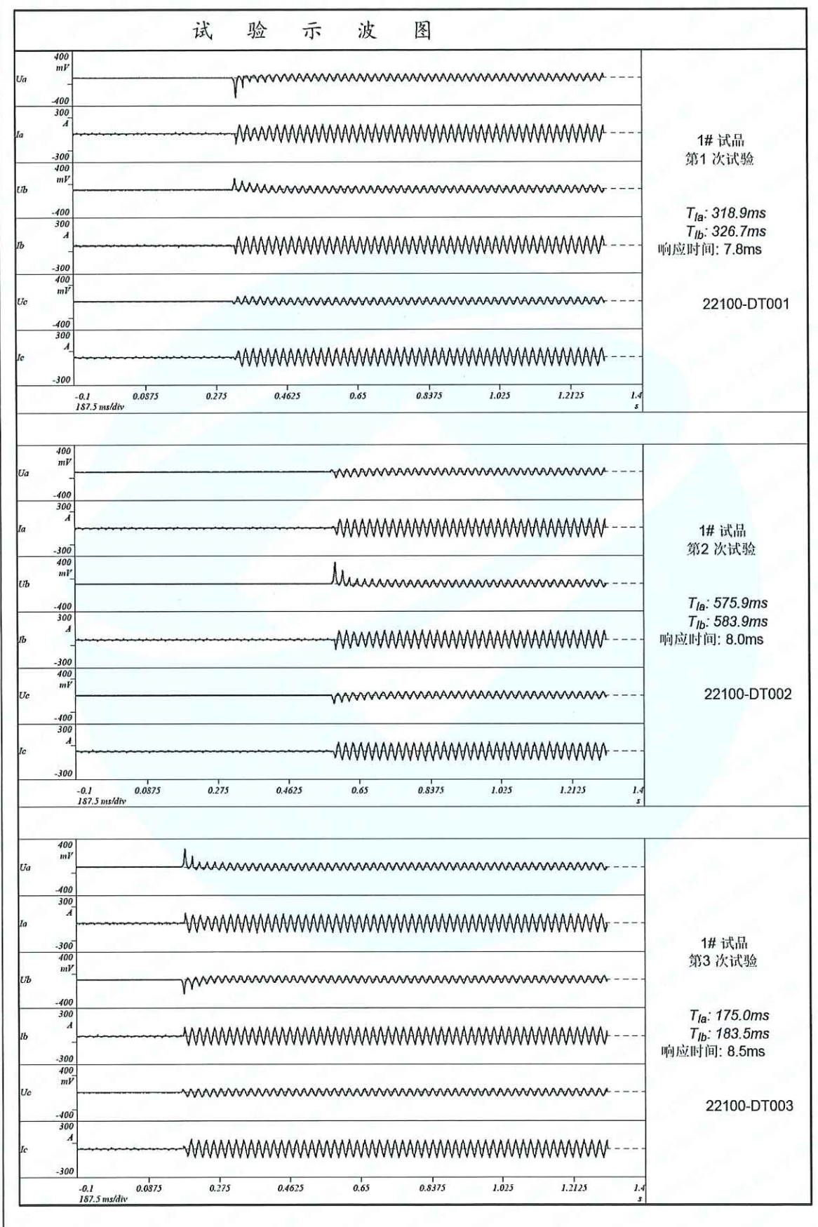
附图 10.20.3 电容器动态响应时间试验示波图
