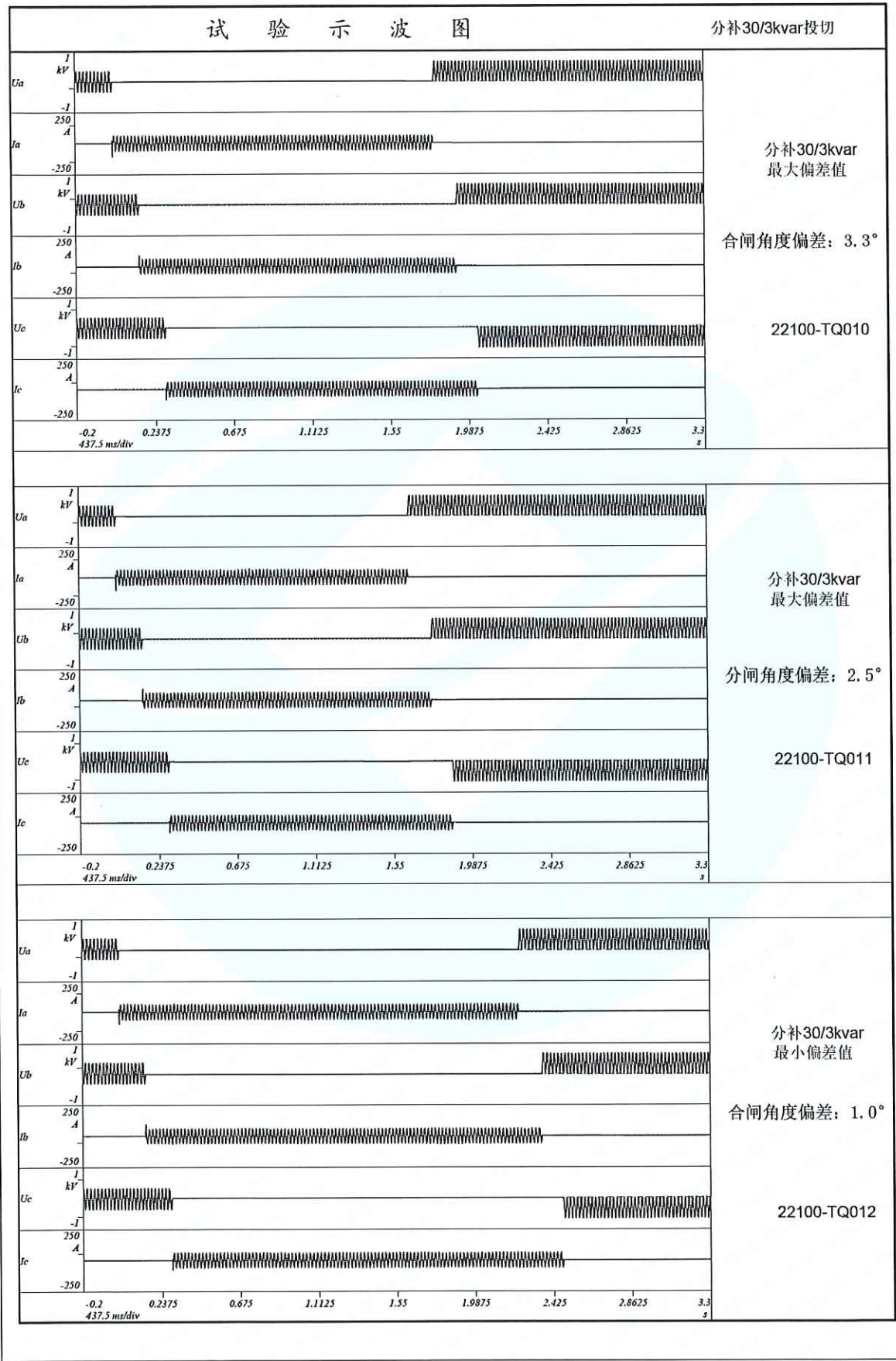
分补 30/3kvar 电容器示波图
