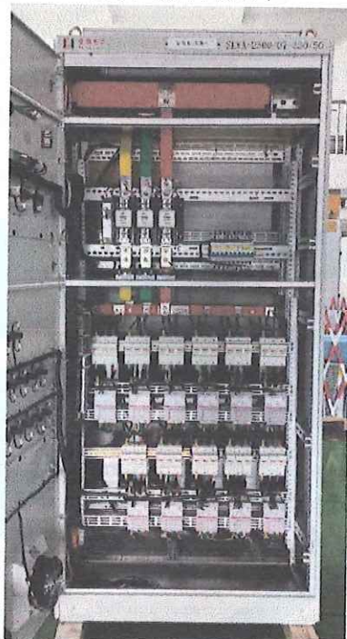
打开前门照片
