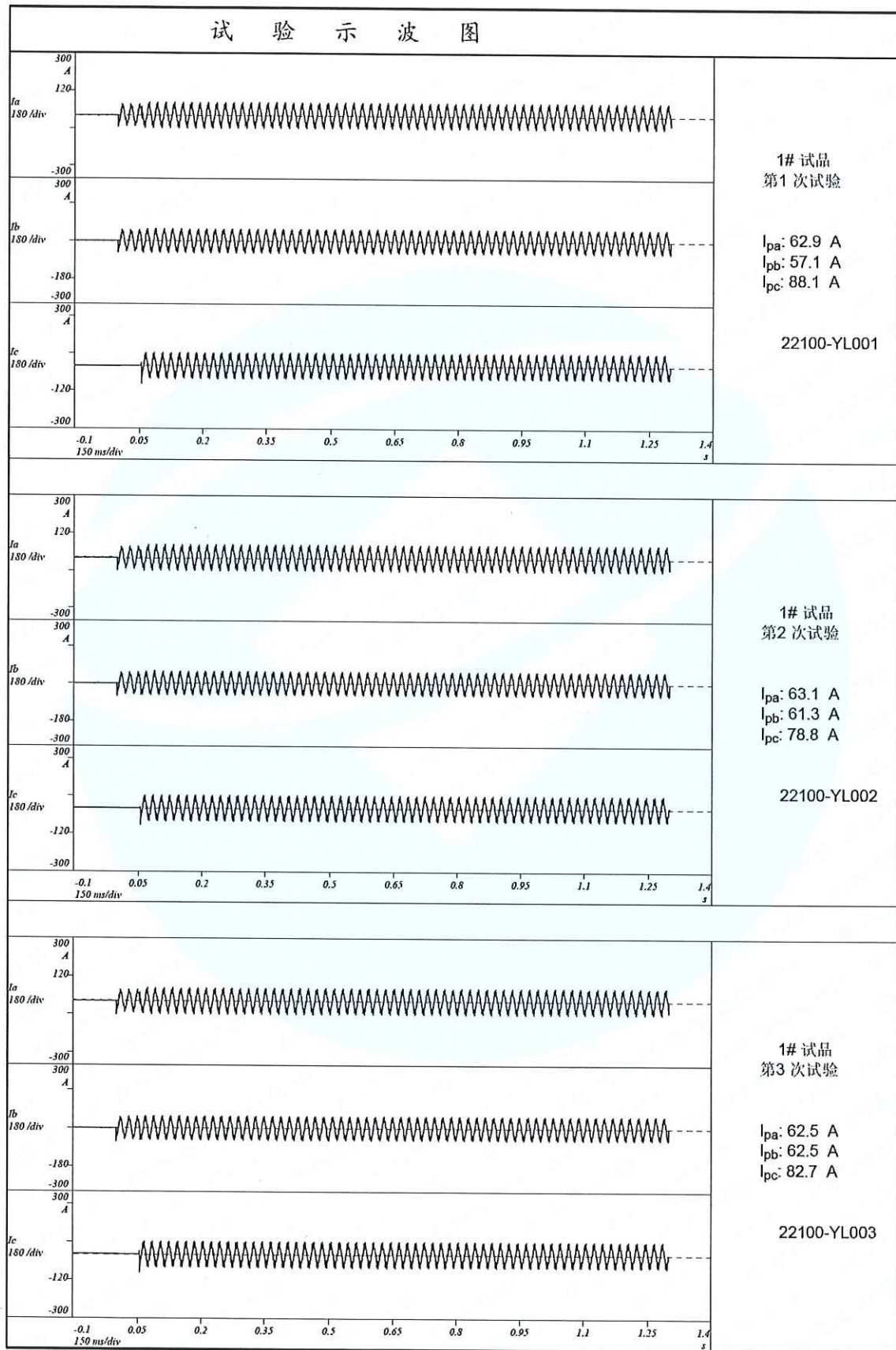
附图 9.15.3 电容器涌流试验示波图
