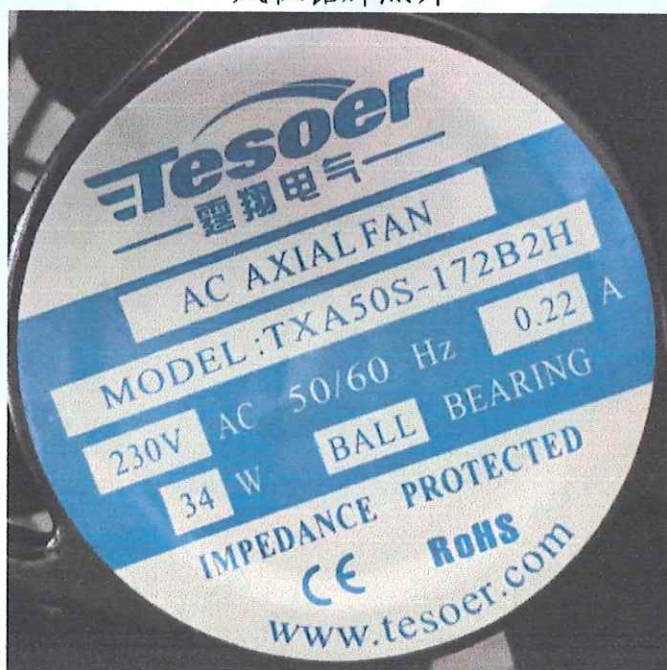
风机铭牌照片
