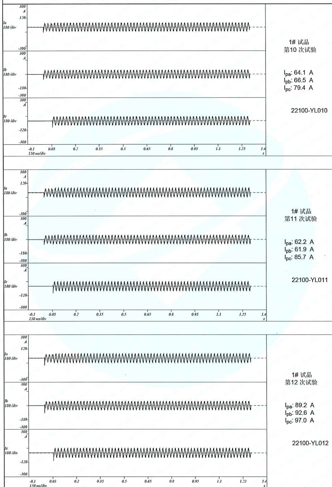
试 验 示 波 图
