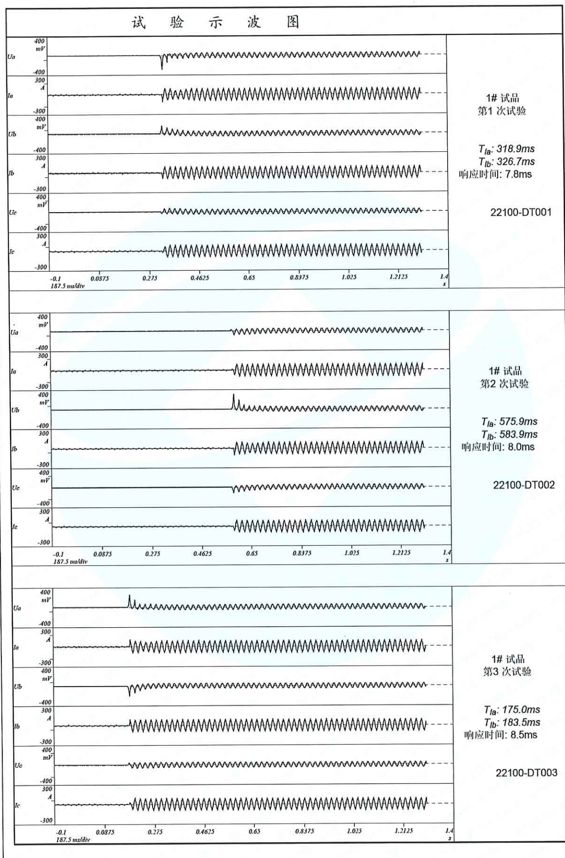
附图 9.17 电容器动态响应时间试验示波图
