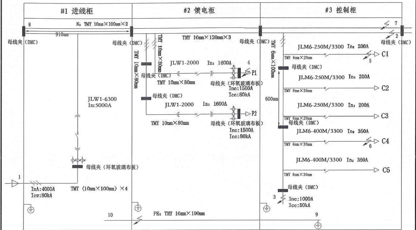
短路试验及绝缘支撑件示意图 DL197421001
