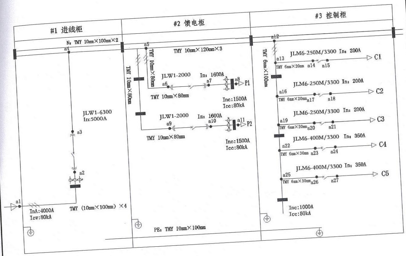
温升试验示意图 WS197421001
