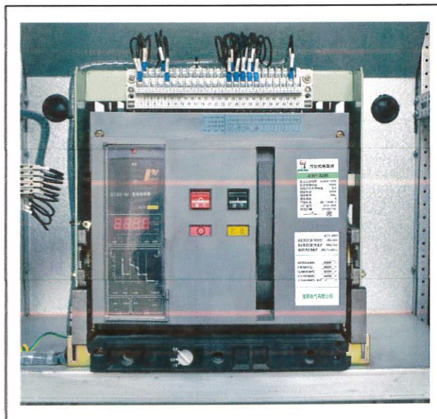
主开关
