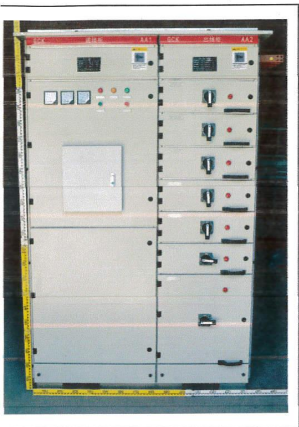
正面
