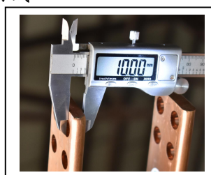
水平母线
