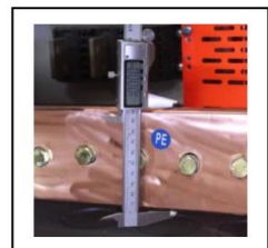
PE 母线
