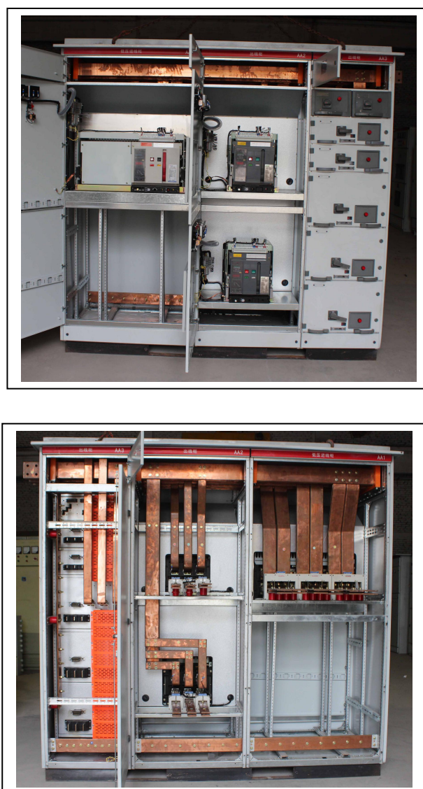
内部结构
