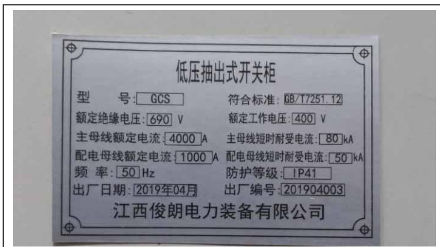
铭牌
