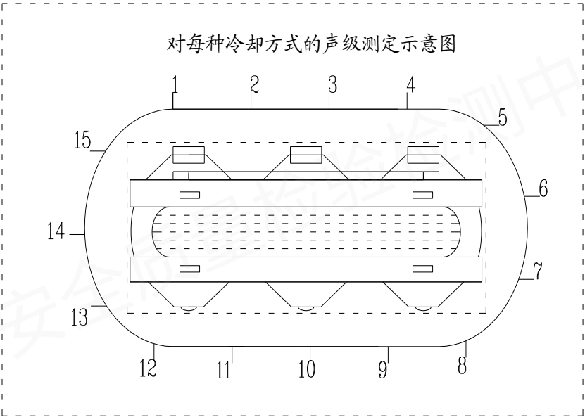
预装式变电站声级测定示意图
